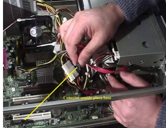
Fig. 13-5 Conector sonido CD-ROM
