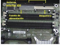
Fig 8. Conectores internos
