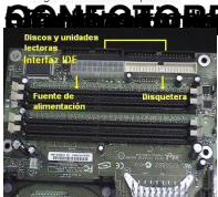
Fig 8 Conectores internos
