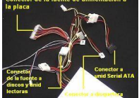
Fig 9 Conectores de la fuente a la placa base
