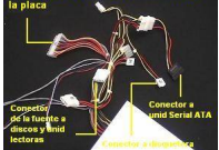
Fig 9 Conectores de la fuente a la placa base
