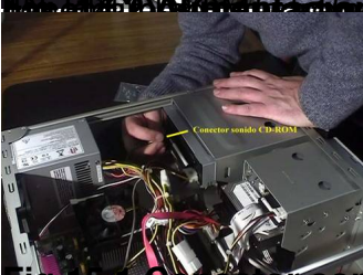
Fig. 13-5 Instalación de CD-ROM
